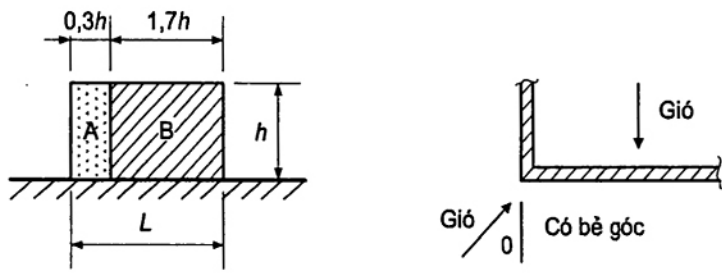
Hình F.1 – Các vùng trên tường phẳng, hàng rào và kết cấu tương tự
