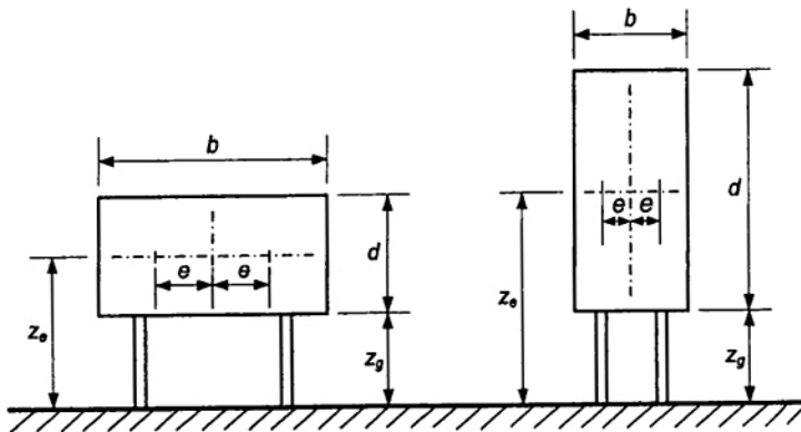
Hình F.2 – Bảng quảng cáo
