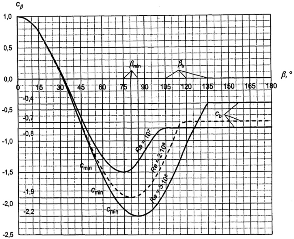
Hình F.19 – Sự phân bố hệ số c_p trên bề mặt trụ tròn
