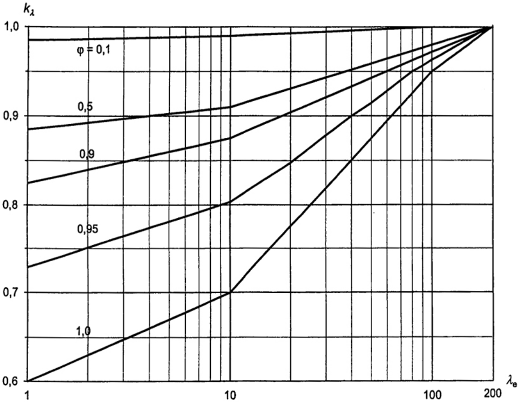
Hình F.27 – Hệ số k_1
