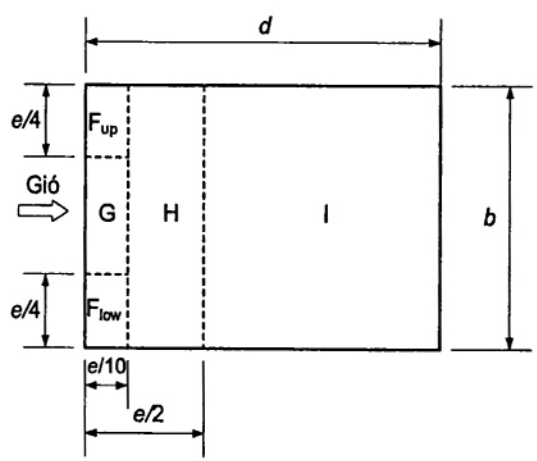
c) Góc hướng gió \theta = 90^\circ
