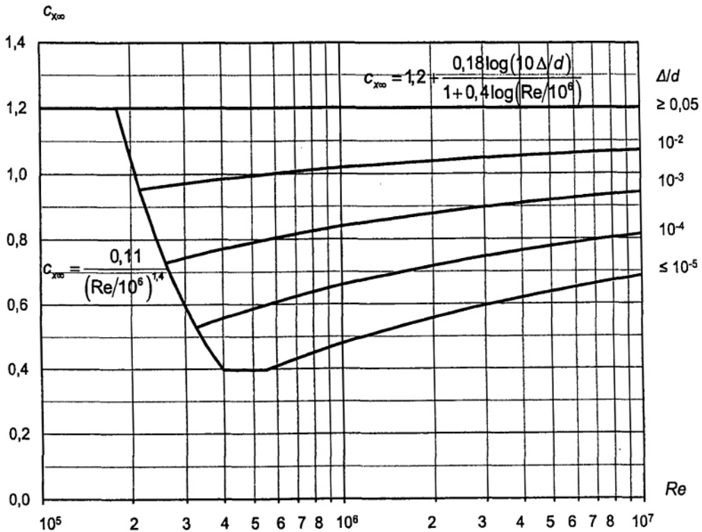
Hình F.20 – Hệ số c_{x00}
