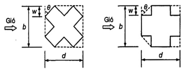
b) Mặt bằng công trình hình chữ X
